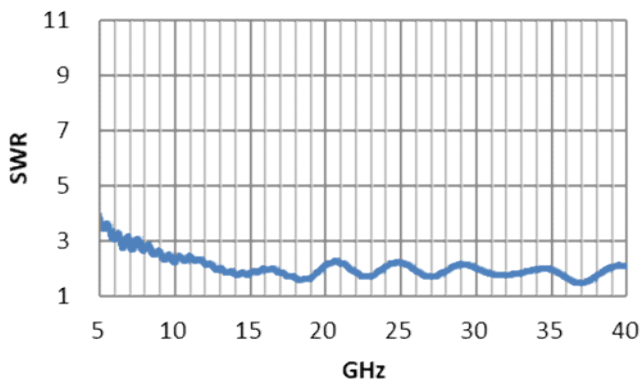
SWR(typ.)
